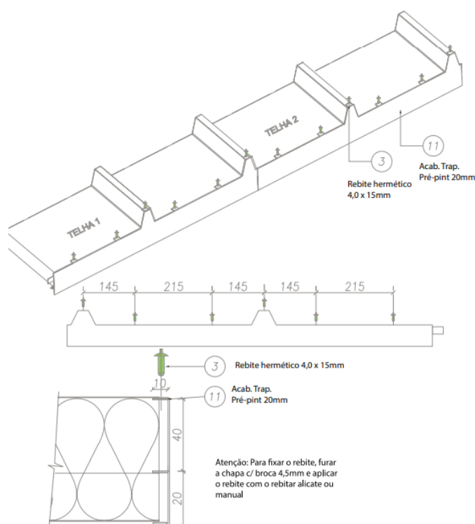
Figura 6-Figura 8-Recomendação do acabamento lateral da telha termoacústica.
