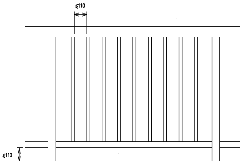
Figura 8- Distância máxima entre perfis de guarda-corpos (gradis).
