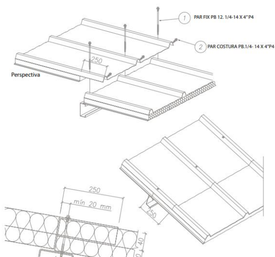
Figura 7-Figura 9-Recomendação do Transpasse da telha termoacústica.
